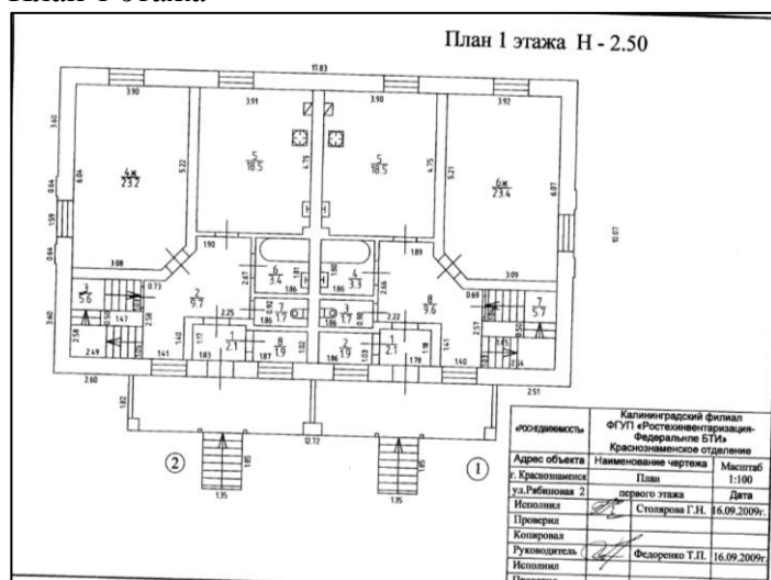
План 1 этажа
