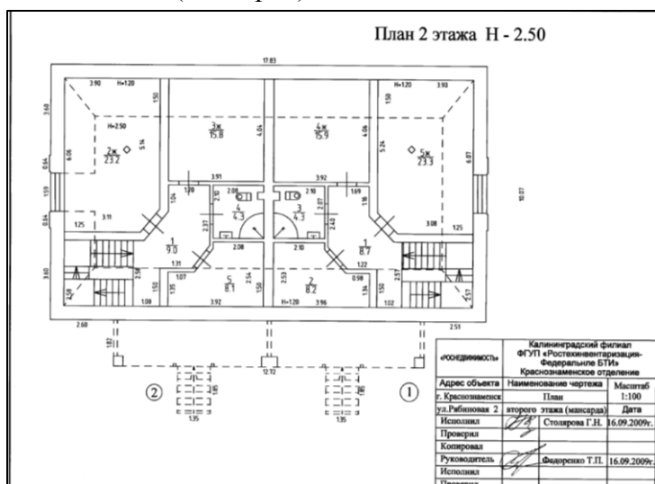
План 2 этажа (мансарда)
